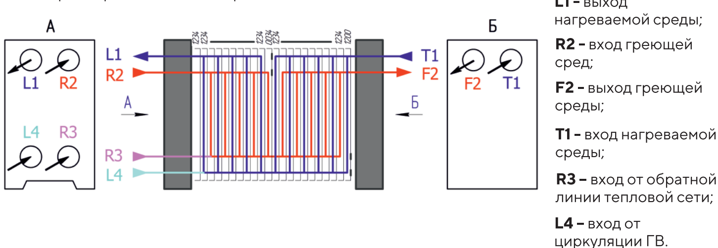
Рис. №4. Принципиальная диаграмма компоновки пакета пластин моноблочного теплообменника с верхним подключением
