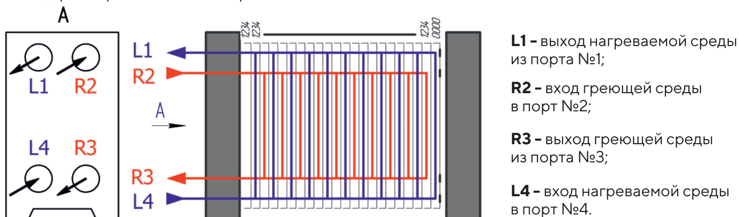
Рис. №2. Принципиальная диаграмма компоновки пакета пластин
